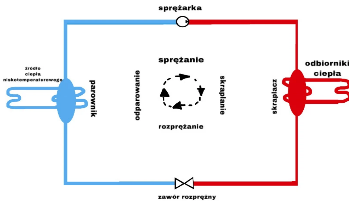
SCHEMAT DZIAŁANIA POMPY CIEPŁA
